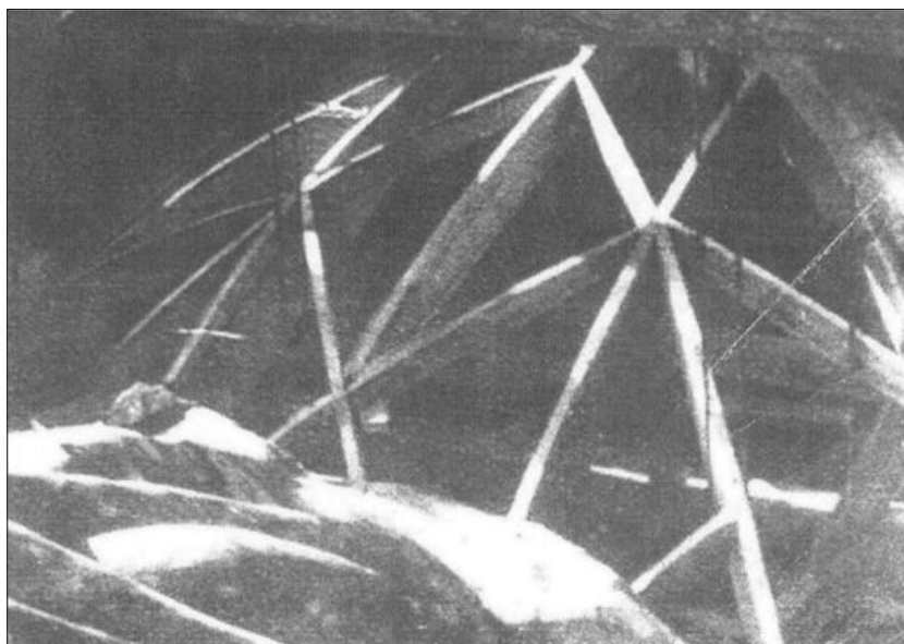
Fot. 44. Krążyny pod odbudowę sklepienia kryształowego w kościele NMP w Gdańsku (fot. J. Tajchman)
