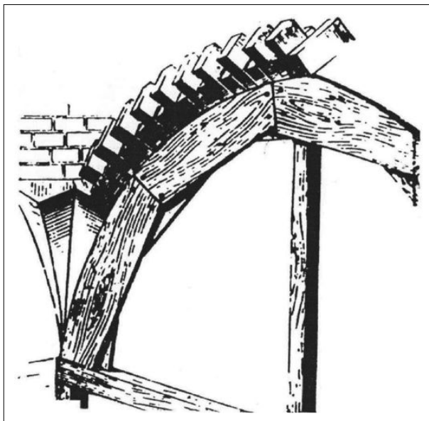
Rys. 47. Zasada budowy sklepienia kryształowego (rys. J. Tajchman)
