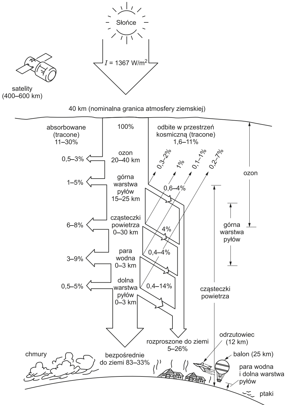
Rys. 1.3. Wpływ atmosfery ziemskiej na światło słoneczne; na podstawie [9]
